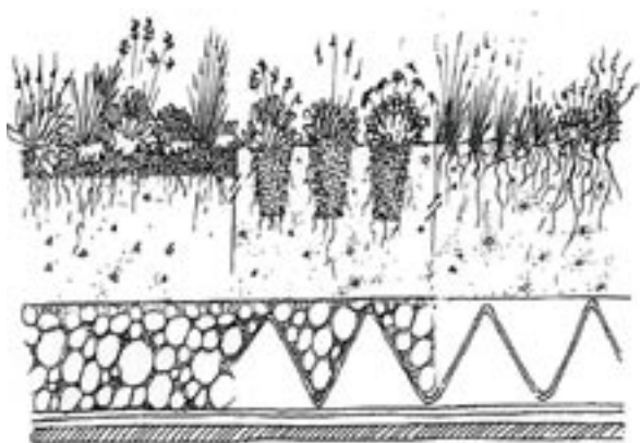
Coupe type d'un toit végétalisé où se superposent la strate végétale, une membrane filtrante, la couche de drainage (agglomérés, ou modules de plastique remplis ou non d'agglomérés), une membrane anti-racine et enfin une membrane d'étanchéité
