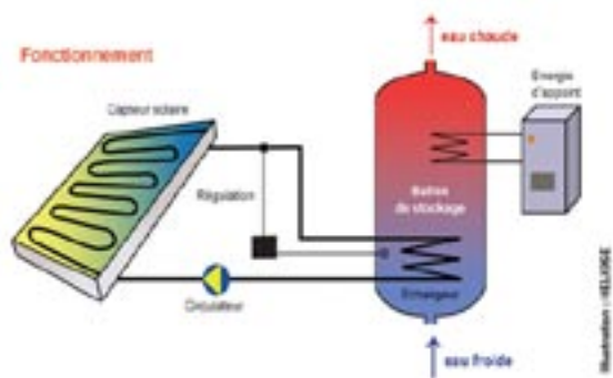
Chauffe-eau solaire à éléments séparés avec appoint indépendant (modèle avec circulation forcée).
