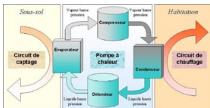
Schéma du principe de fonctionnement d'une pompe à chaleur
