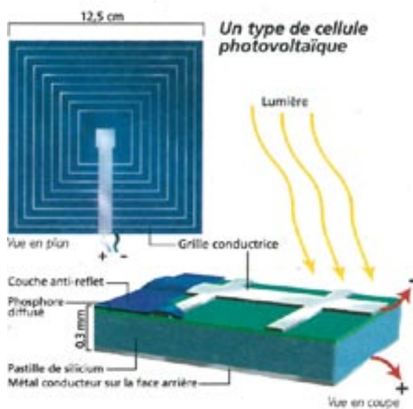
Principe de fonctionnement d'une cellule solaire photovoltaïque
